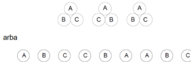
3 pav. Fazių išdėstymas grupėje
