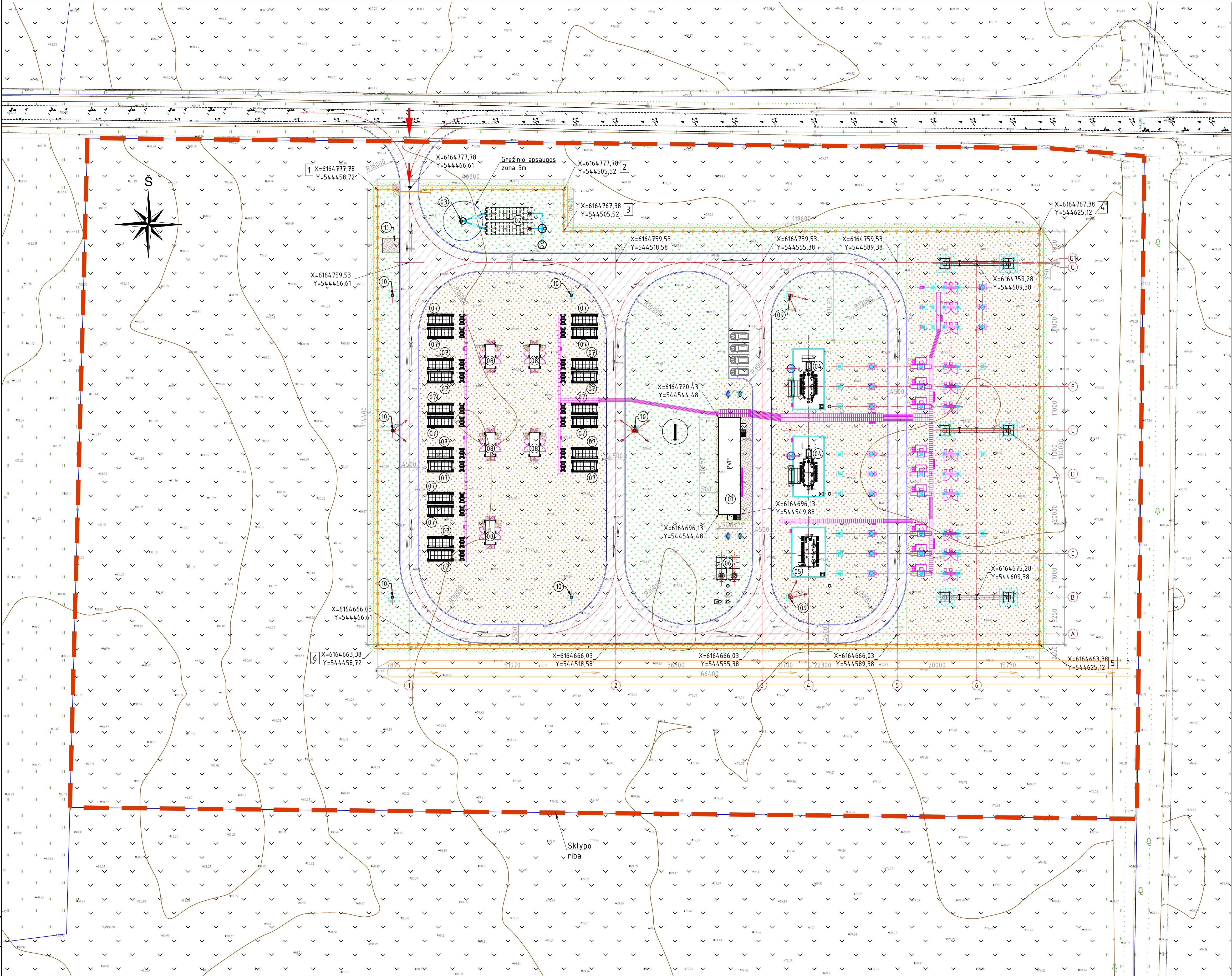
Sklypo ir aplinkotvarkos planas. M1:500
