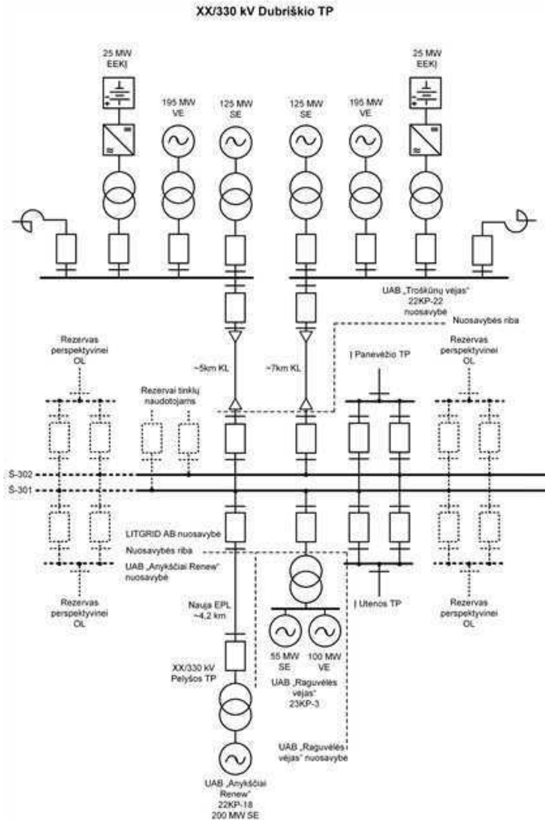
1 schema. Planuojamų elektrinių prijungimo prie elektros perdavimo tinklo principinė schema.
