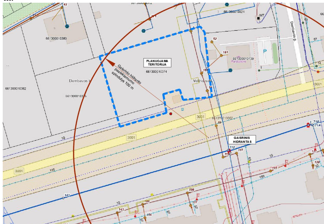
2 pav. Gaisrinio hidranto, šulinio Nr. 112, pasiekiamumo spindulys 100 m, inžinerinių tinklų žemėlapyje pagrindu.
